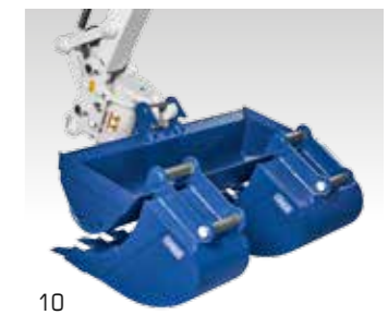
10 SYMLOCK MIT TRANSPORTKLINGE
